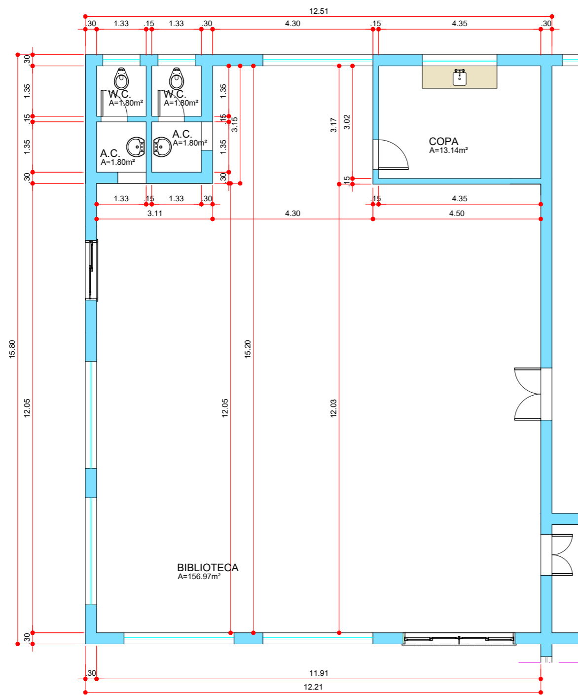
PLANTA ESC. 1:100
