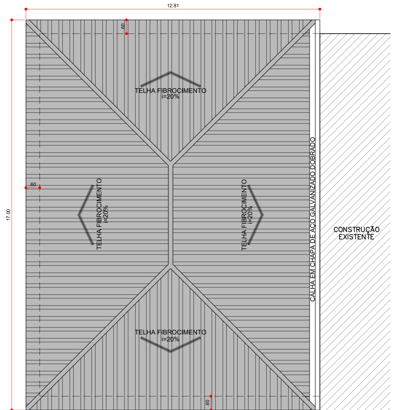
VISTA DA COBERTURA ESC. 1:100
