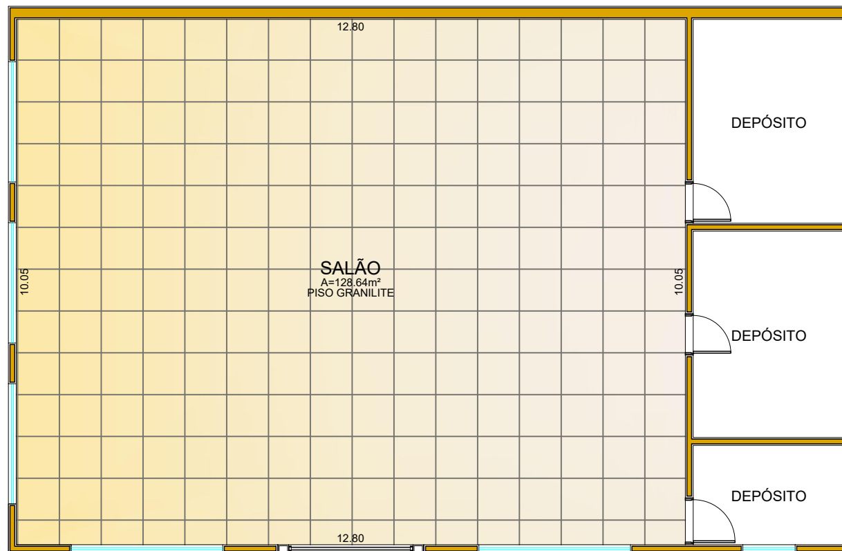
PLANTA ESC. 1:100
